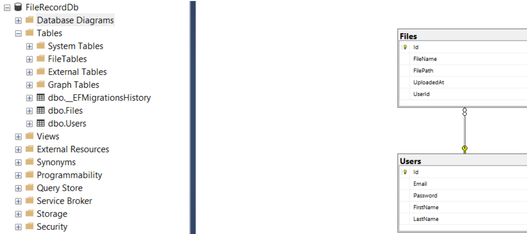
Şekil 8.11 SQL Server'daki ilişkili iki ana tablo
